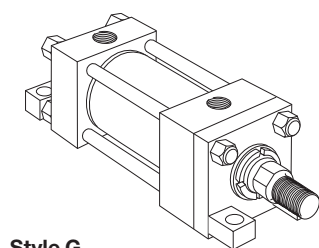
Style G Side End Lug (NFPA Style MS7)
